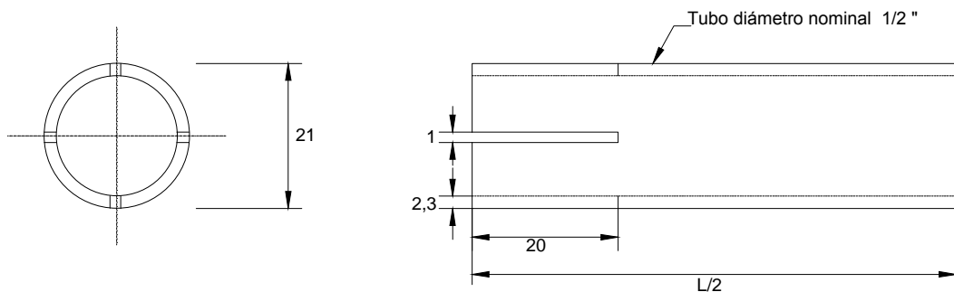
BUJE
