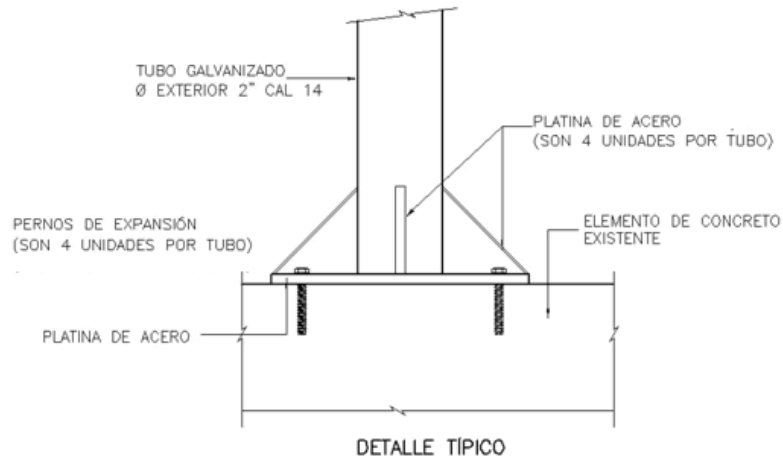
Esquema 1. Detalle anclajes de barandas de seguridad en obras de EPM
