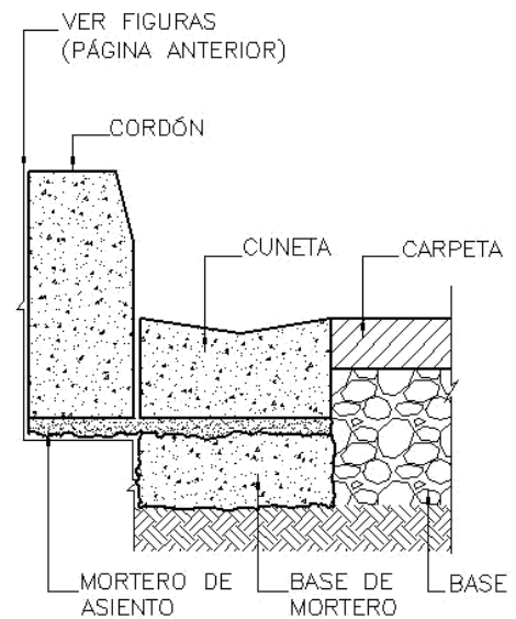
f. CUNETAS SOBRE BASE DE MORTERO.
