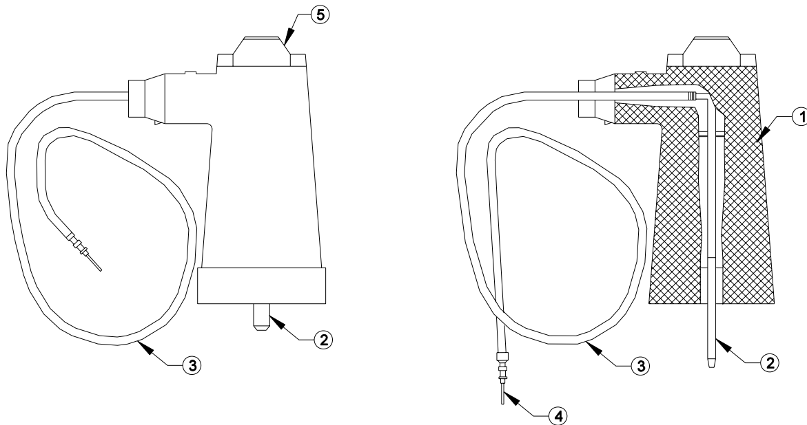
CONECTOR DE COBRE TIPO PIN
