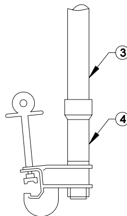
CONECTOR TIPO GRAPA
