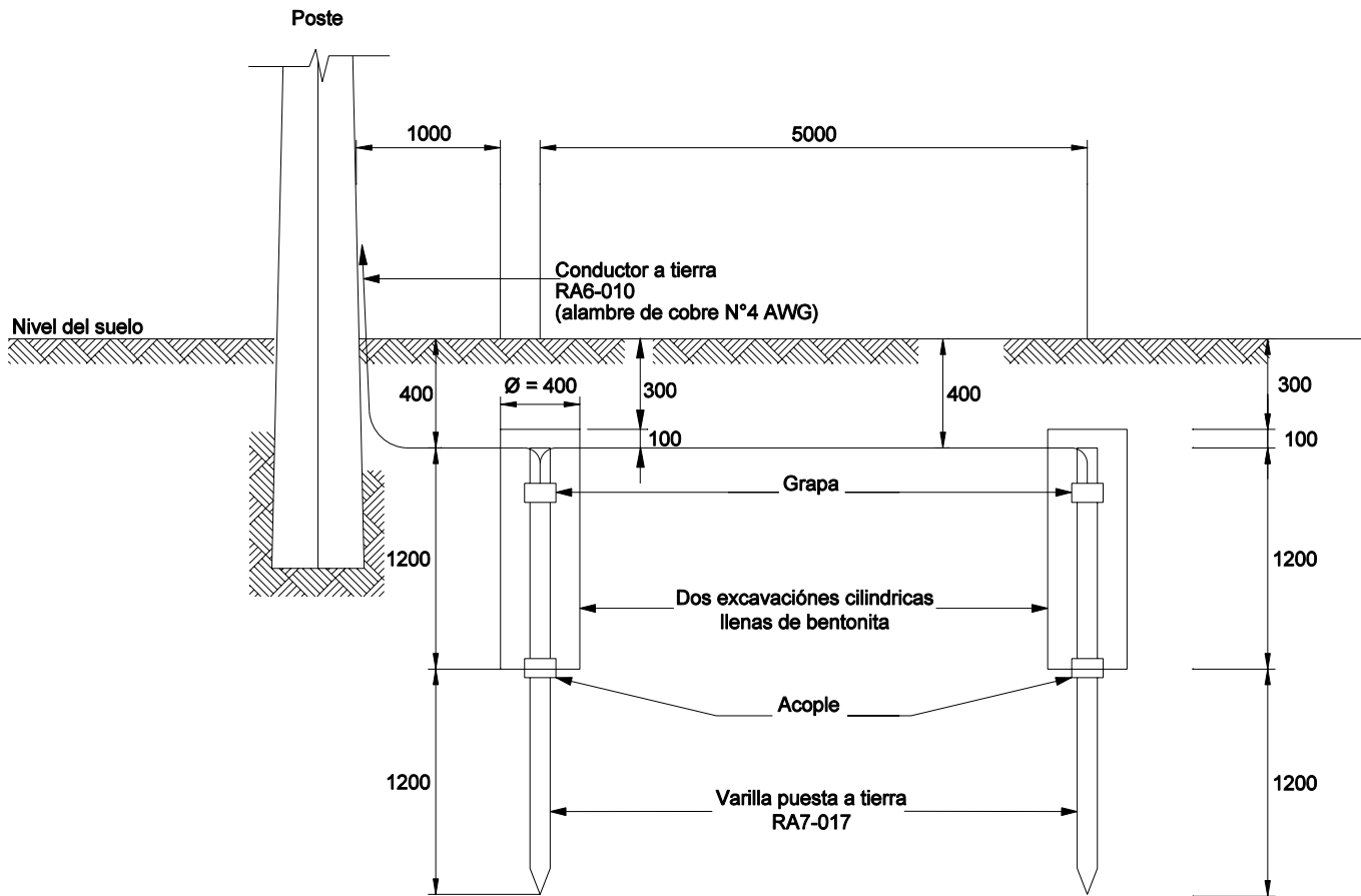
CORTE A - A (VER FIGURA 3)
