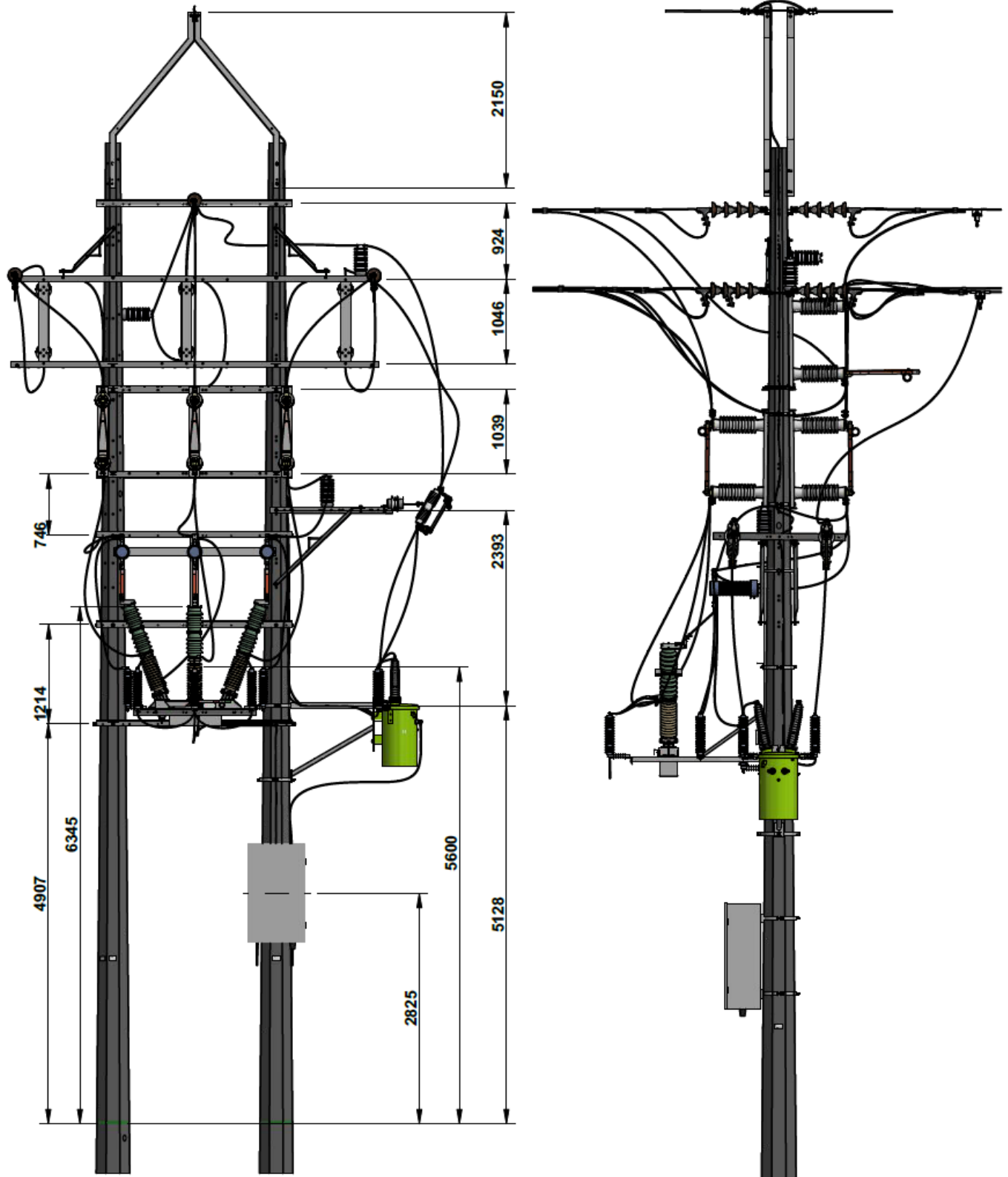
Figura 33. Vista principal y dimensiones - Instalación de reconector trifásico 44 kV
