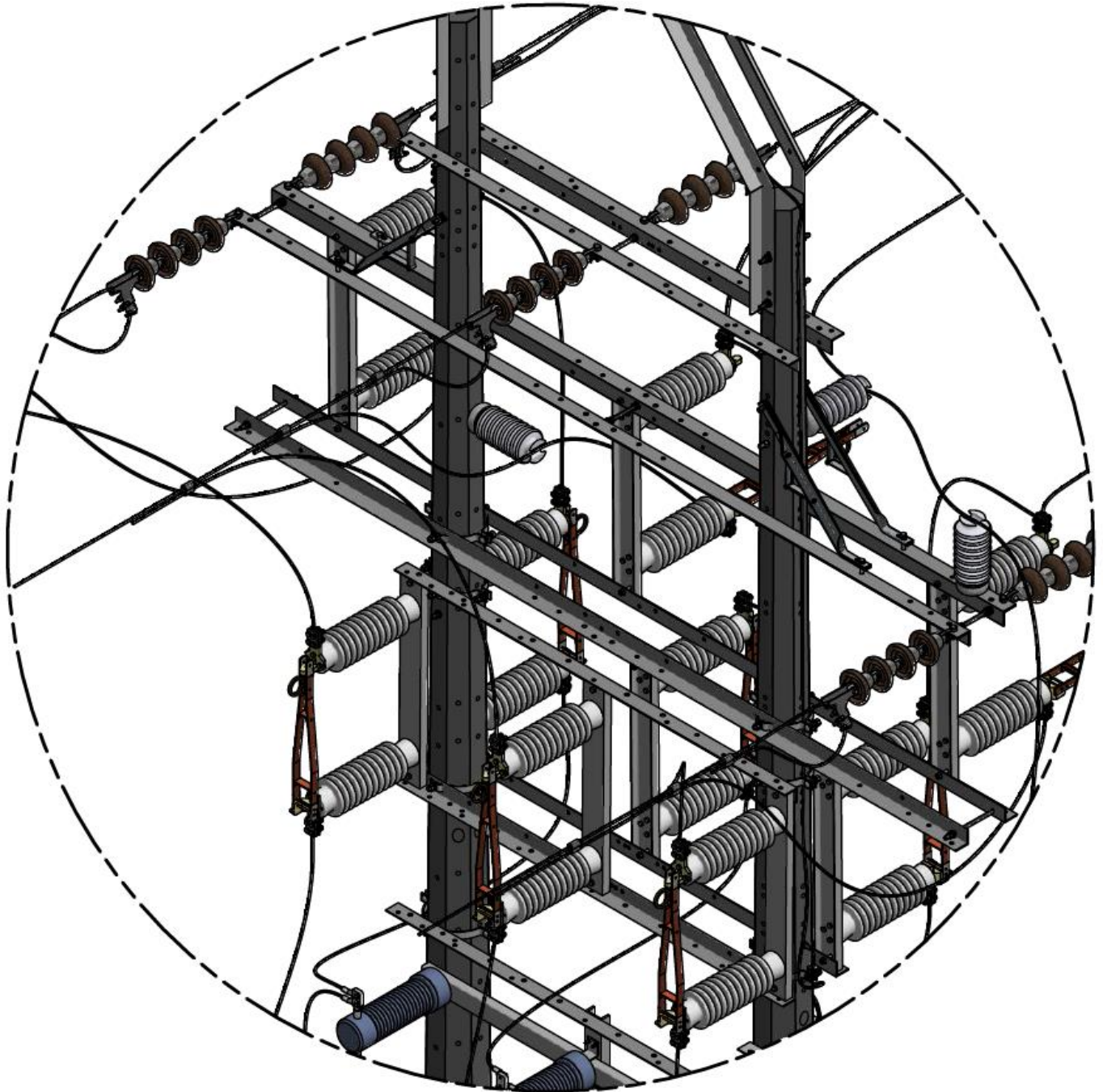
Figura 34. Detalle montaje By-pass y Seccionamiento - Instalación de reconector trifásico 44 kV
