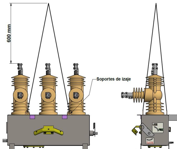
Figura 4. Levantamiento del reconectador para izaje e instalación.
