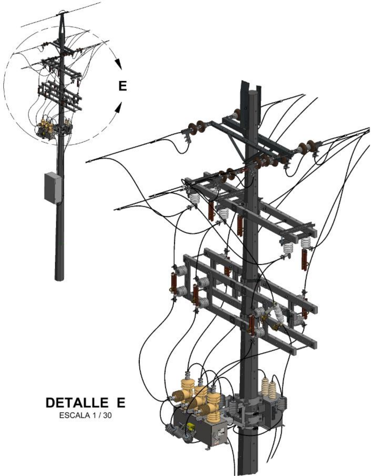
Figura 13. Detalle montaje Bypass y Seccionamiento - Instalación de reconector trifásico en troncal 13.2 kV – Línea Viva
