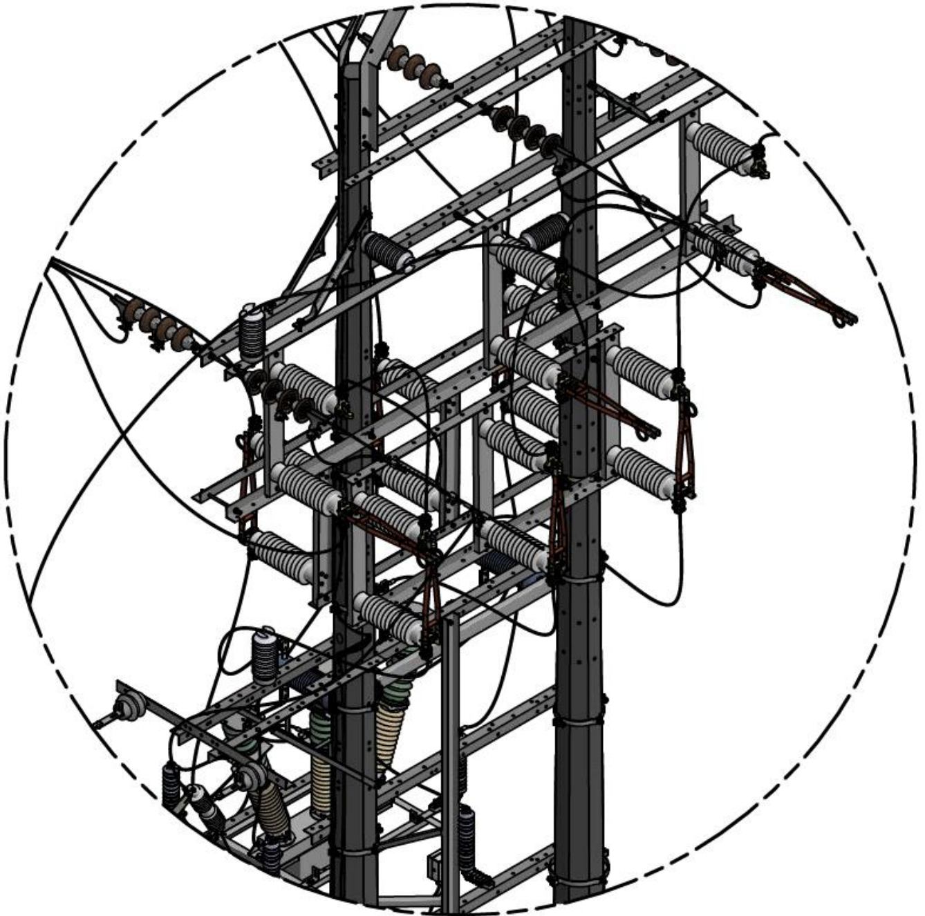
Figura 35. Detalle montaje By-pass y Seccionamiento - Instalación de reconector trifásico 44 kV
