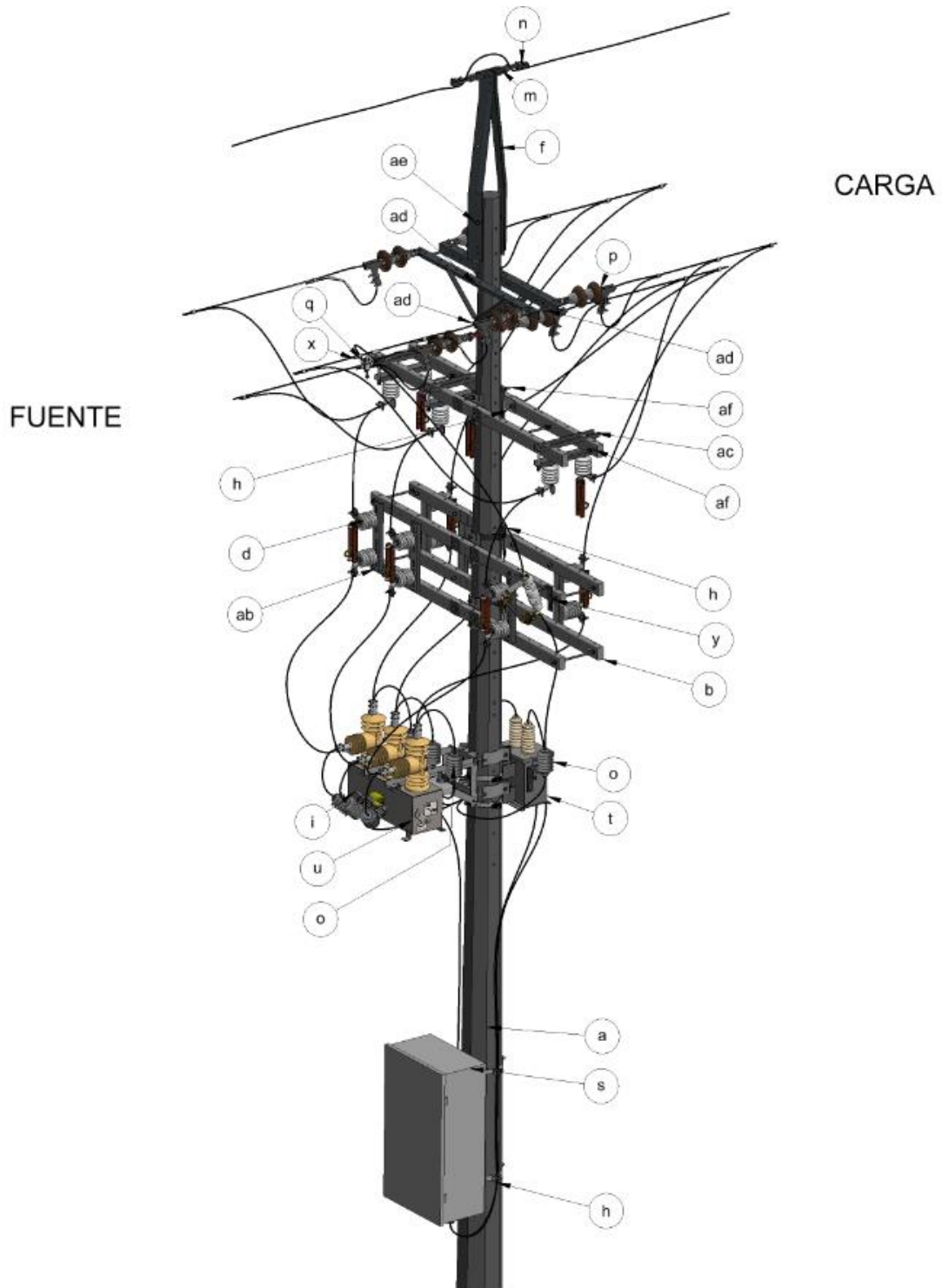
Figura 11. Isométrico - Instalación de reconvertador trifásico en troncal 13.2 kV – Línea Viva
