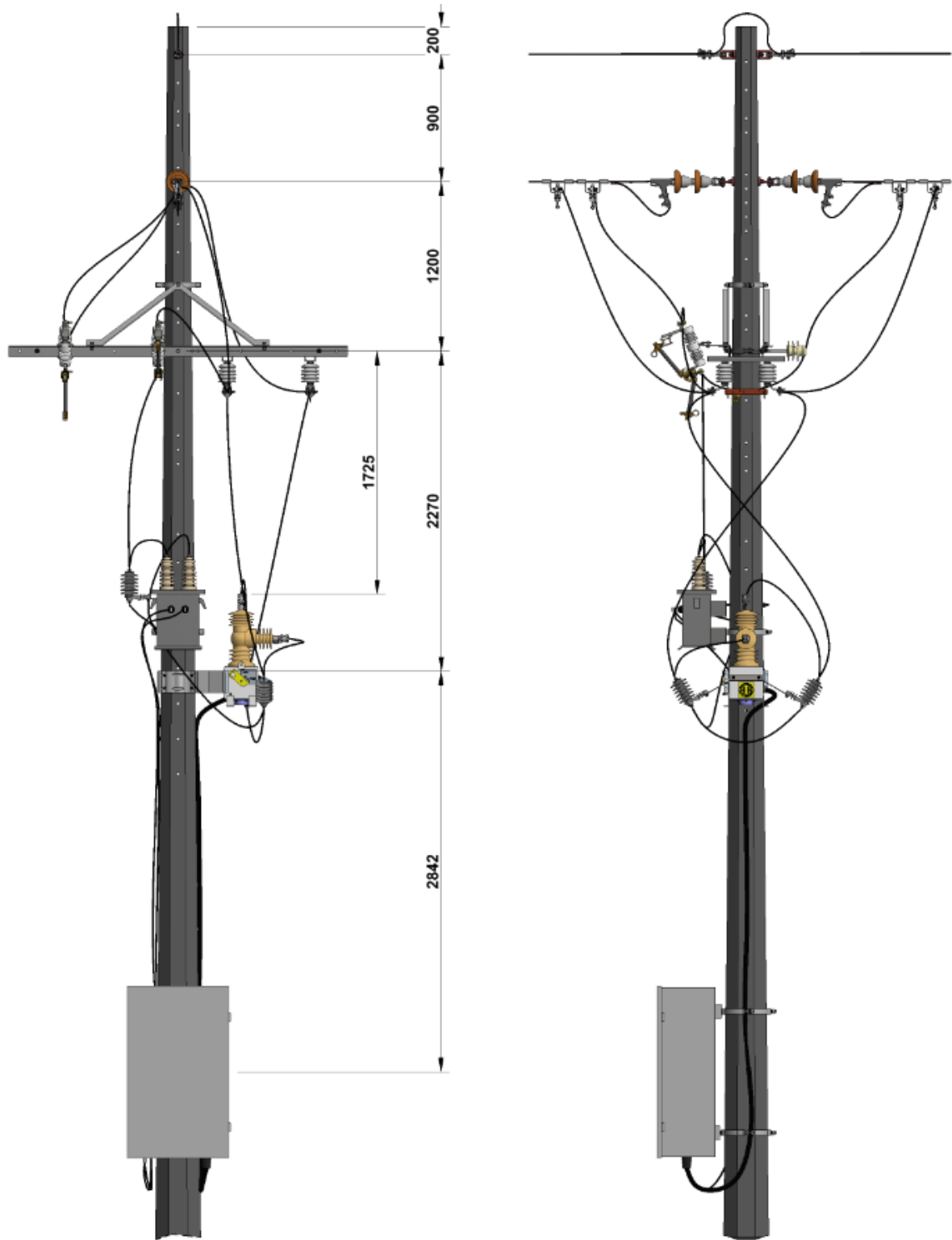
Figura 30. Vista principal y dimensiones - Instalación de reconectador monofásico 7.62 kV
