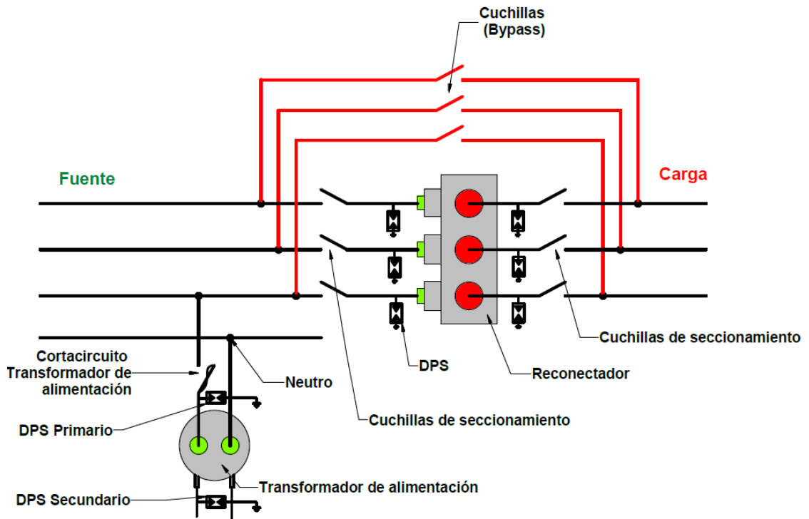
Figura 9. Diagrama unifilar – Instalación reconector trifásico en ramal
