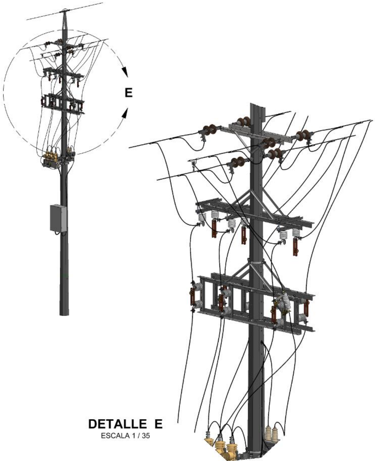
Figura 16. Detalle montaje Bypass y Seccionamiento - Instalación de reconector trifásico en troncal 13.2 kV – Línea Muerta
