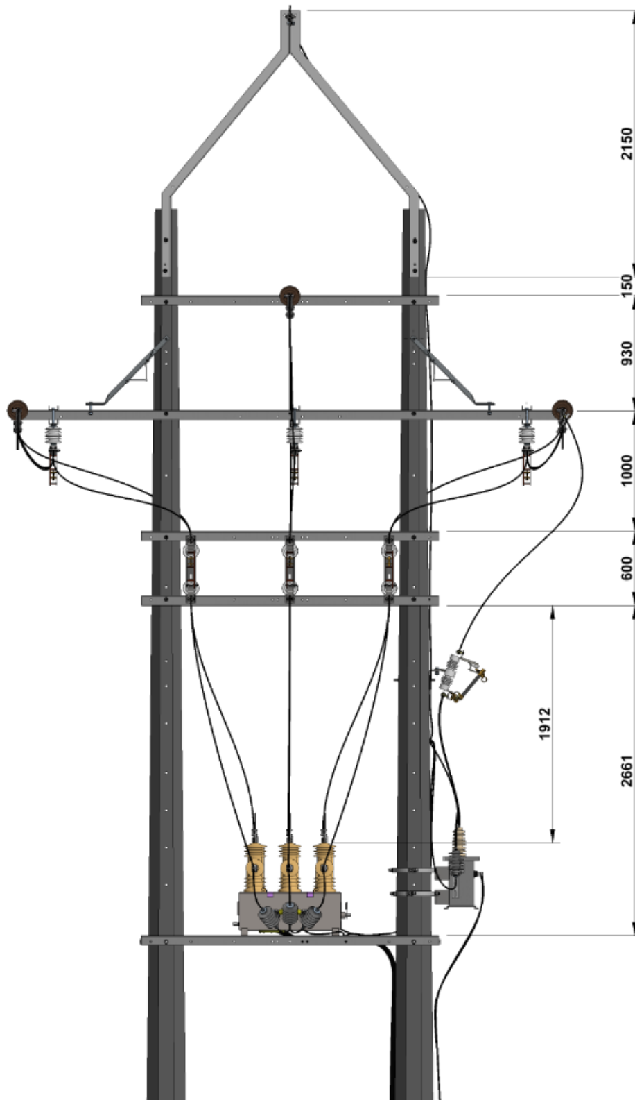
Figura 26. Vista principal y dimensiones - Instalación de reconector trifásico 13.2 kV en estructura tipo H
