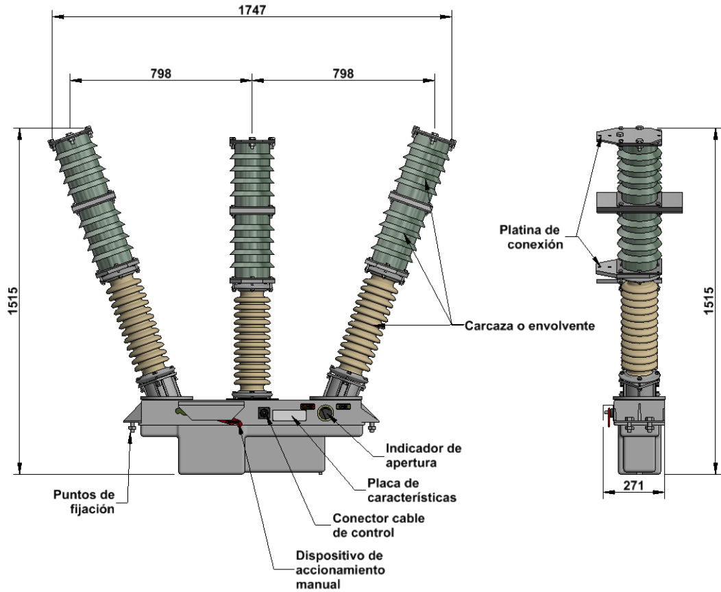
Figura 40. Reconnectador Trifásico Joslyn 44 kV
