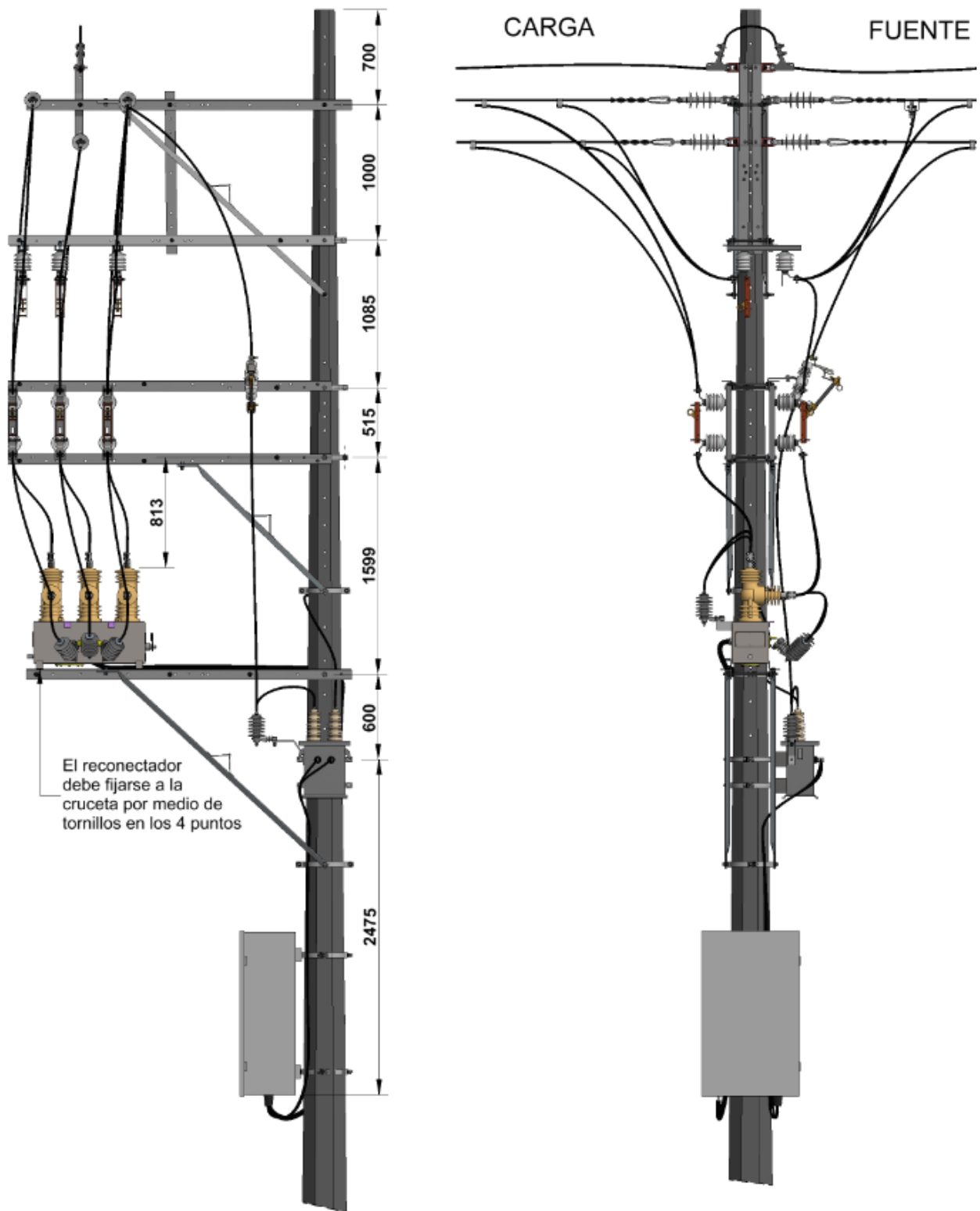
Figura 23. Vista principal y dimensiones - Instalación de reconector trifásico 13.2 kV cruceta volada
