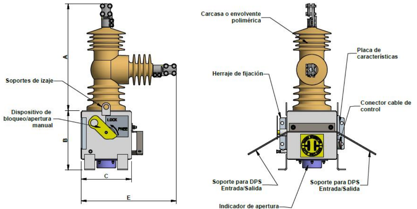
Figura 39. Reconector monofásico ENTEC 7.62 kV
