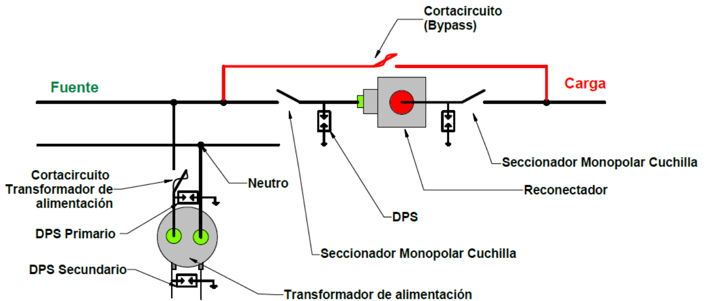
Figura 10. Diagrama unifilar – Instalación reconector monofásico
