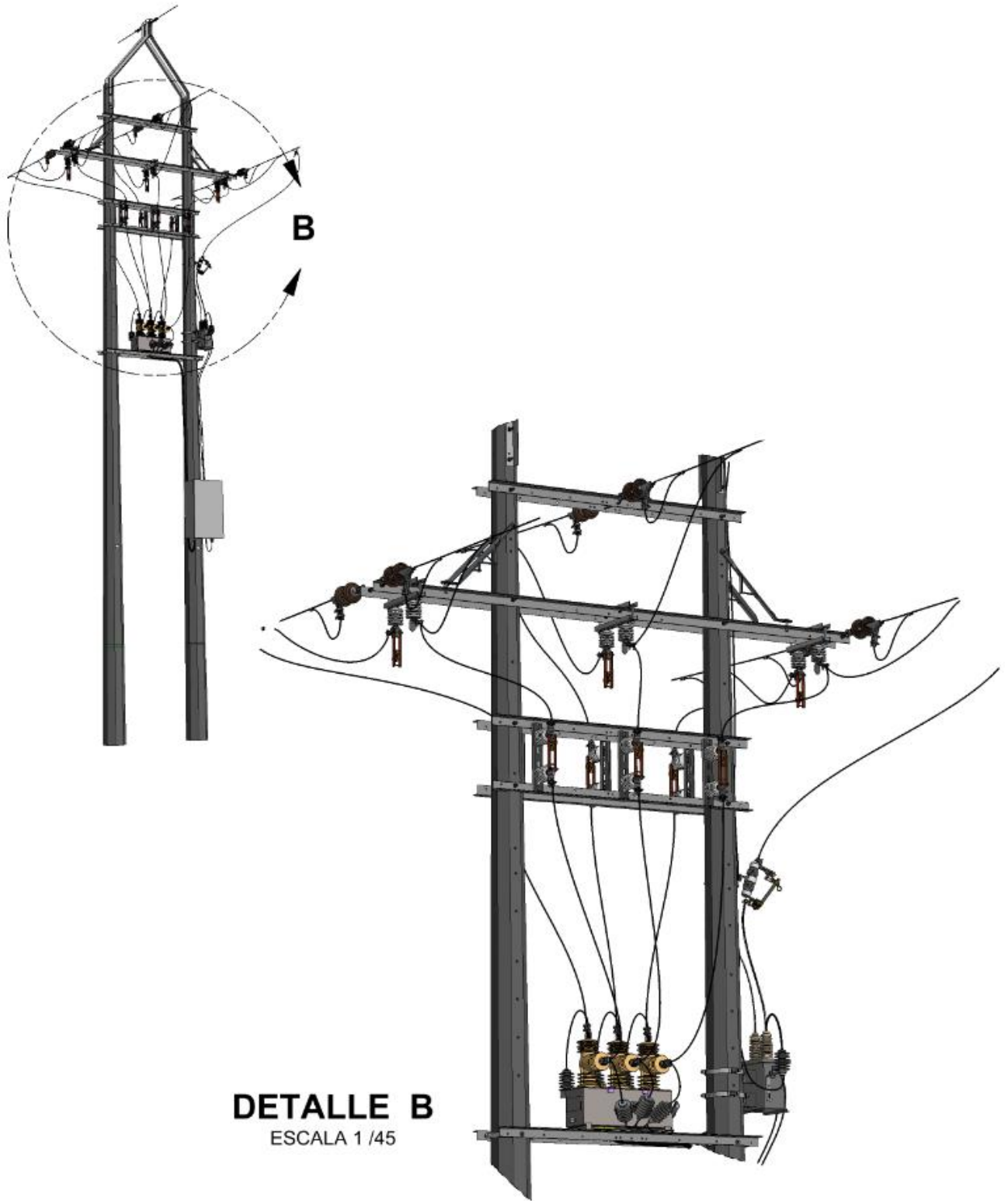
Figura 27. Detalle montaje Bypass y Seccionamiento - Instalación de reconectador trifásico 13.2 kV en estructura tipo H
