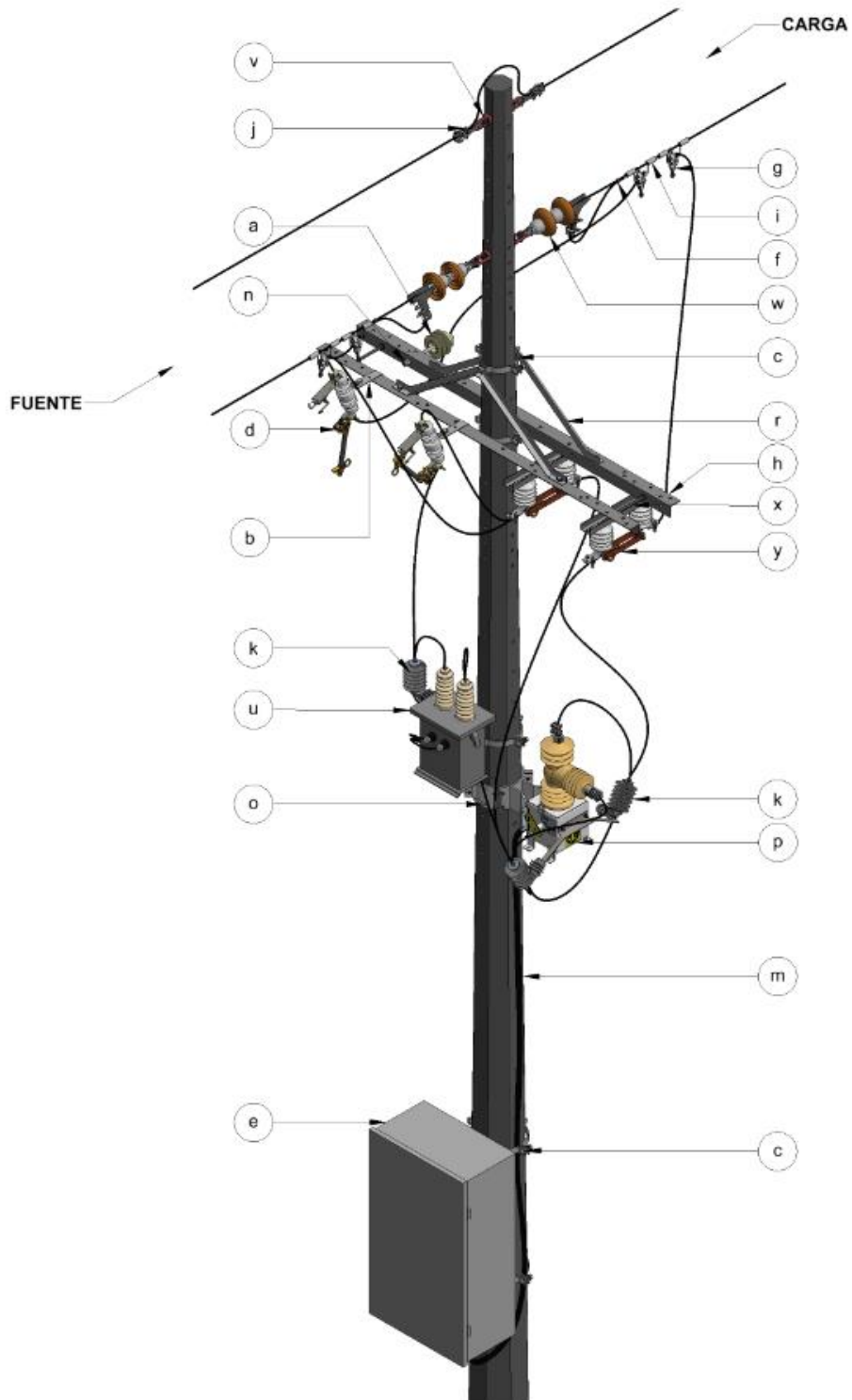
Figura 29. Isométrico - Instalación de reconectador monofásico 7.62 kV
