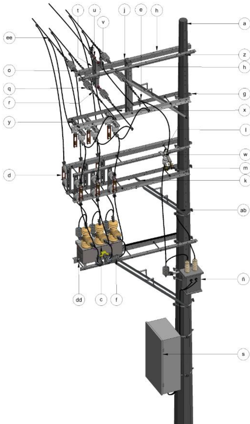
Figura 22. Isométrico - Instalación de reconectador trifásico 13.2 kV cruceta volada
