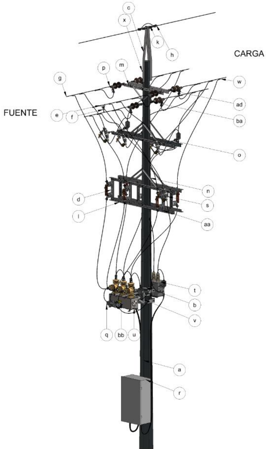
Figura 18. Isométrico - Instalación de reconectador trifásico en ramal 13.2 kV – Línea Muerta
