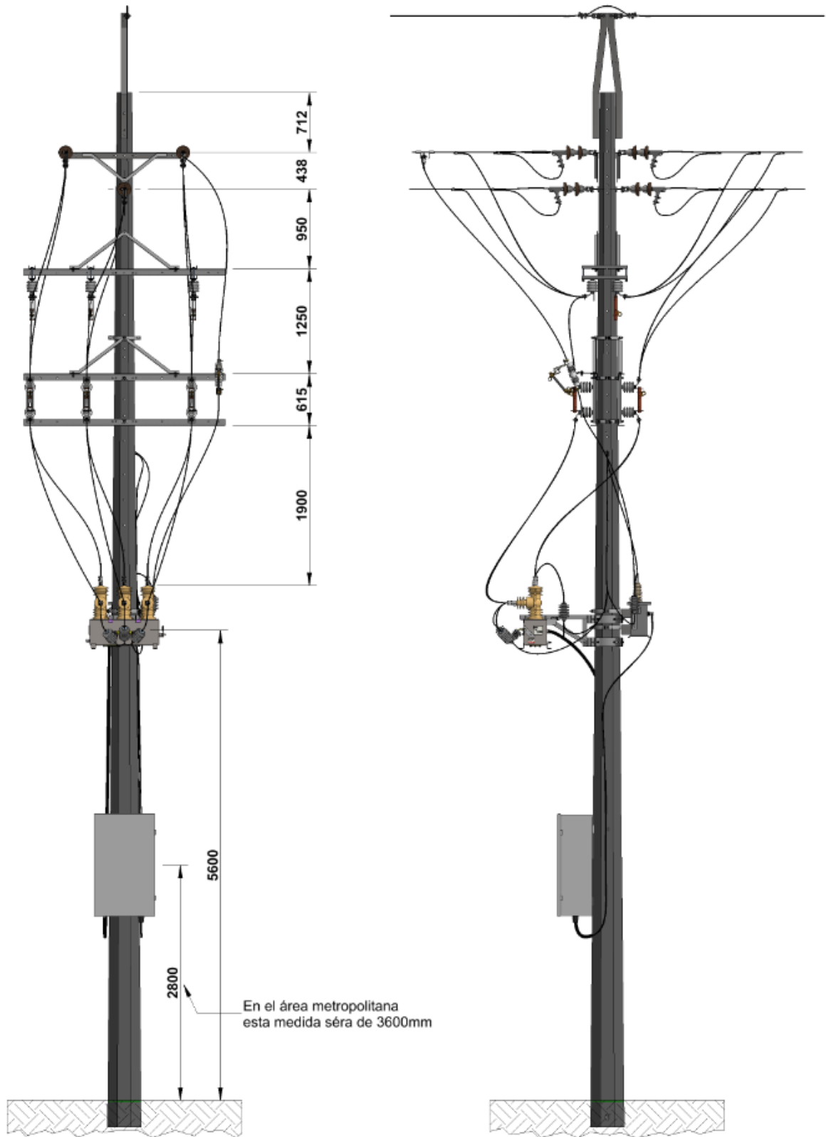
Figura 15. Vista principal y dimensiones - Instalación de reconectador trifásico en troncal 13.2 kV – Línea Muerta
