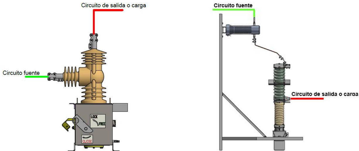
a) Reconectador ENTEC 13.2 kV
