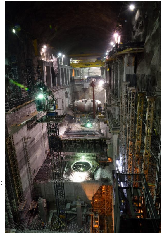
Casa de máquinas: montaje de los equipos (turbinas y generadores).
