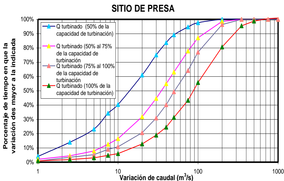
Figura 7.2.30 Porcentaje de variación de caudales en el sitio de presa
