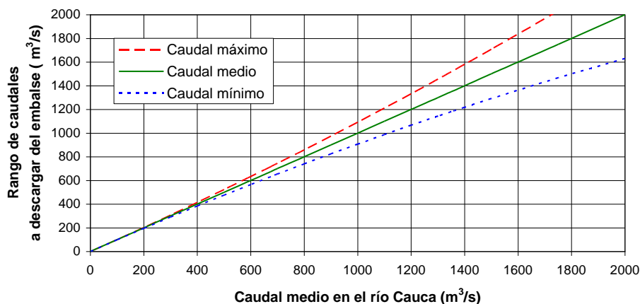
Figura 7.2.31 Restricción de la variación de caudales extremos evacuados por el embalse en un lapso de 24 horas
