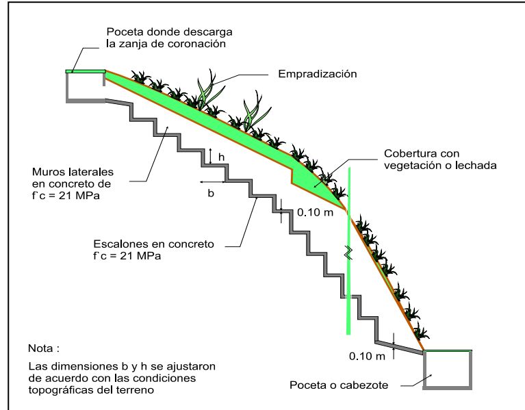
Figura 7.2.26 Disipadores de energía
