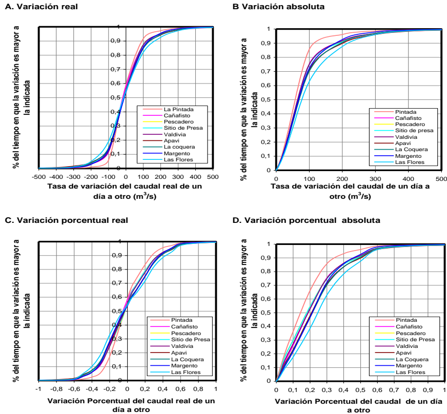
Figura 7.2.29 Variación de caudal de un día a otro
