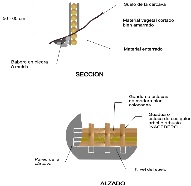
Figura 7.2.27 Modelo de trincho para la protección de pilas de suelo almacenado
