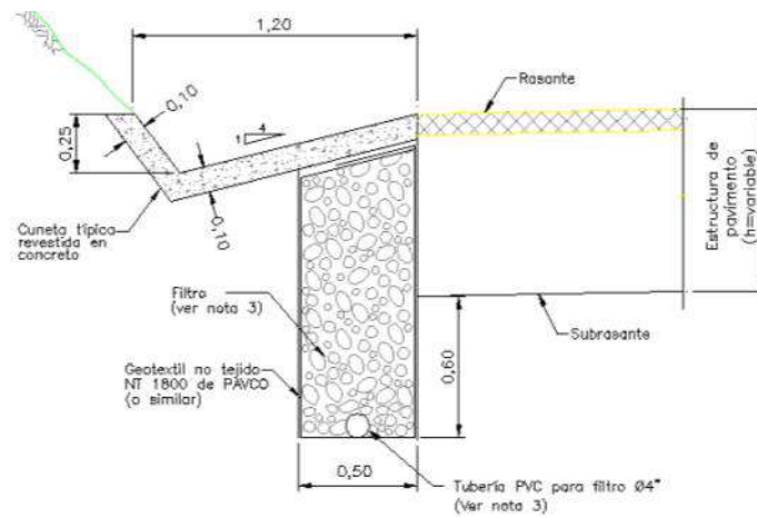
Figura 7.2.10. Cuneta típica y subdrenes en suelo
