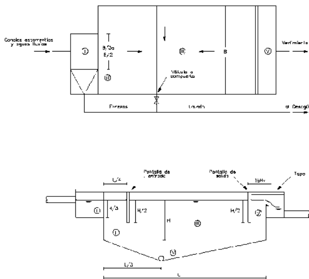
Figura 7.2.23 Esquema típico de sedimentador
