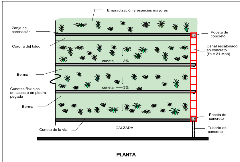
7.2.24 Construcción de bermas cunetas en taludes
