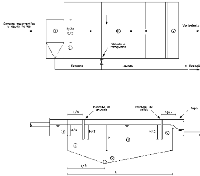
Figura 7.2.2 Esquema típico sedimentador
