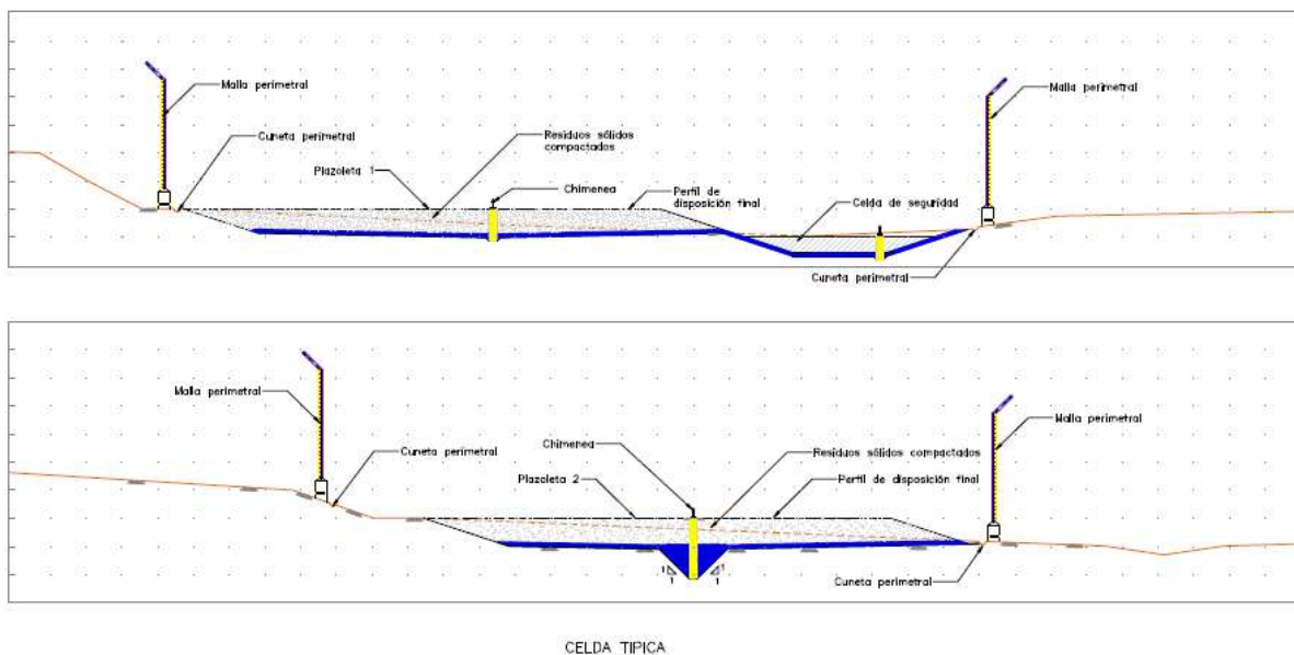
Figura 7.2.16 Esquema típico de una celda de disposición
