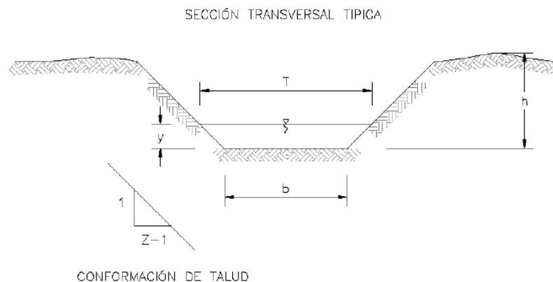
Figura 7.2.5 Esquema recolección de aguas lluvia
