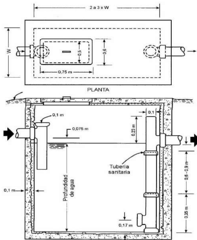
Figura 7.2.3 Esquema trampa de grasas
