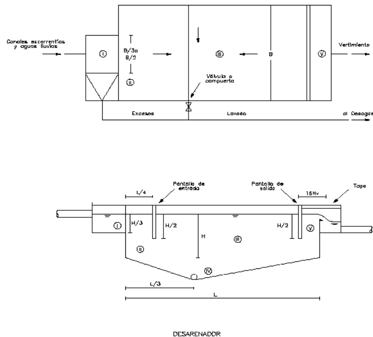
Figura 7.2.4 Esquema sedimentador
