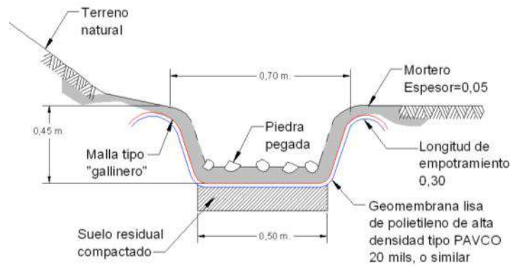
Figura 7.2.9. Cuneta típica en geomembrana y mortero para la ronda de coronación
