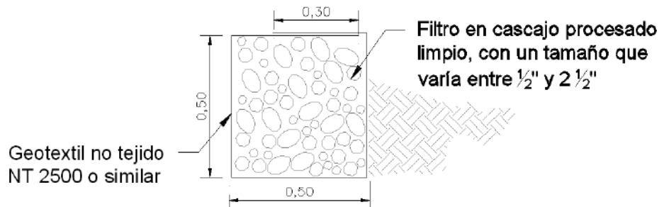
Figura 7.2.15-Filtro típico para el relleno
