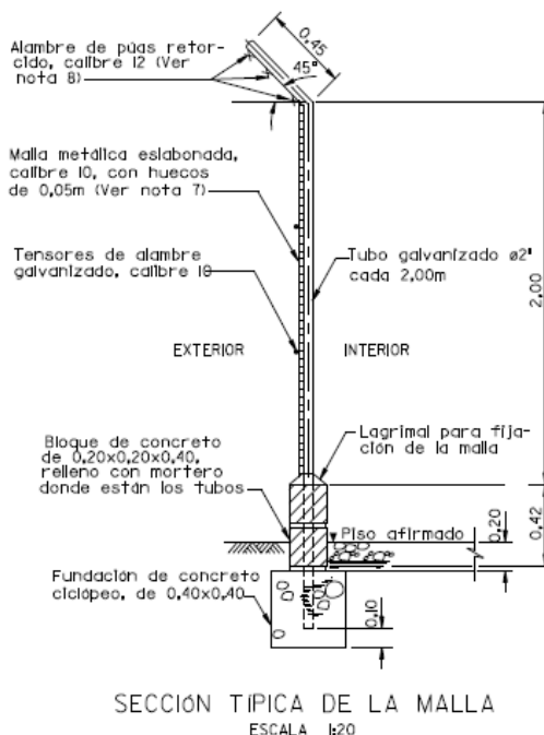
Figura 7.2.8 Esquema típico de cerramiento
