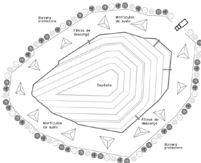
Figura 7.2.28 Disposición y protección de suelo en los depósitos del Proyecto Hidroeléctrico Ituango
