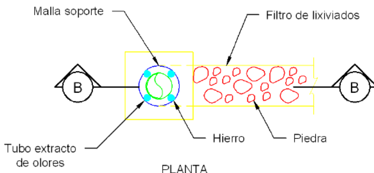
Figura 7.2.13. Vista en planta de chimenea de gases
