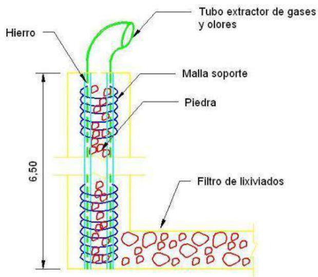
SECCION "B-B"
