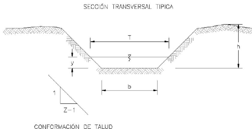
Figura 7.2.22 Sección transversal típica para canales perimetrales
