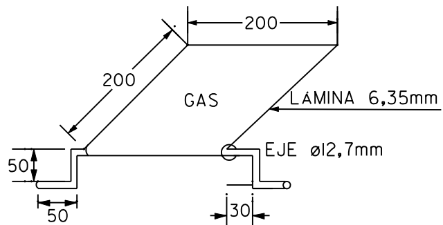
DETALLE DE TAPA METALICA PARTE INTERIOR
